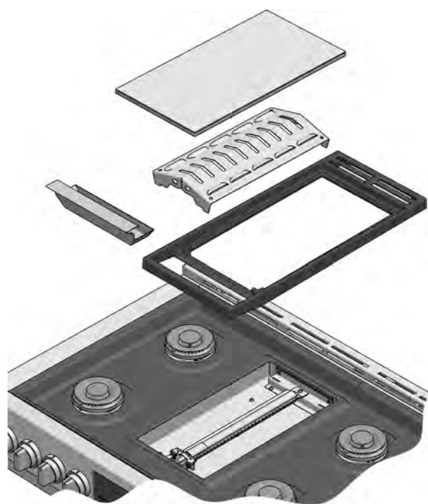
VISTA DETALLADA DE LA REJILLA DEL QUEMADOR
