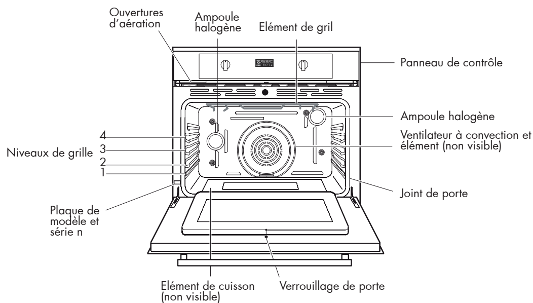
Arrière de la grille du four
