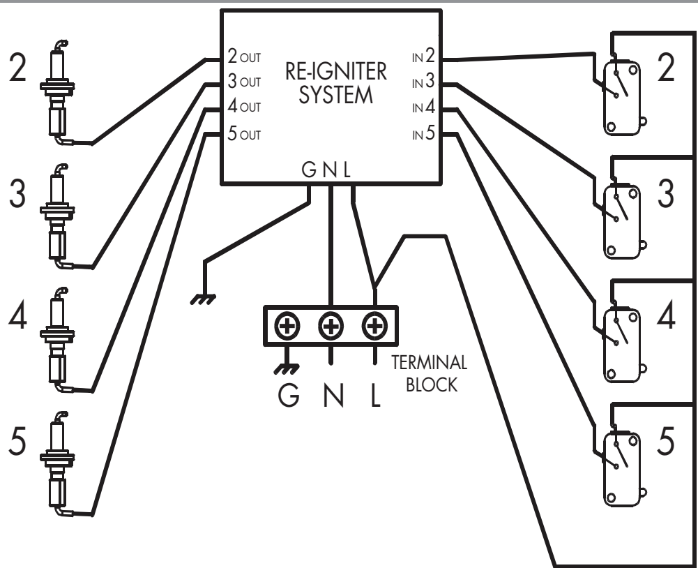
DIAGRAMA ELÉCTRICO (4 ZONAS)
